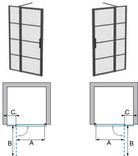
KB17 L Venstrehengslet
